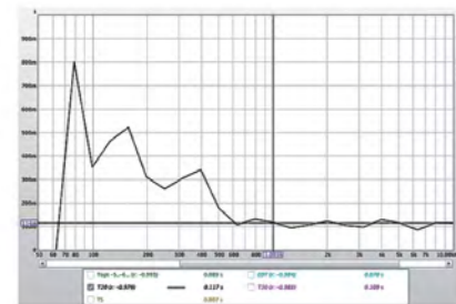
混響時間 Reverberation time
